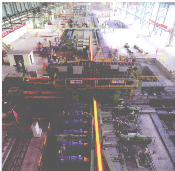
百米高速钢轨万能轧机
