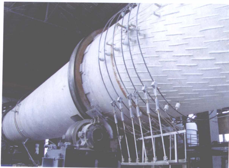
具有国内领先水平的硫酸法钛白生产线
