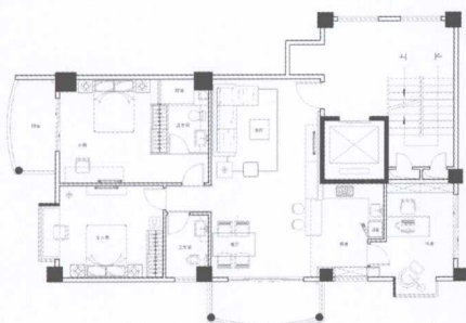
平面布置图 1:100
