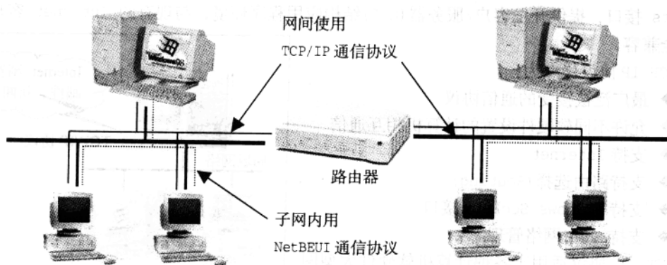
图 1-6 解决 NetBEUI 在广域网中效率低的一种方法
