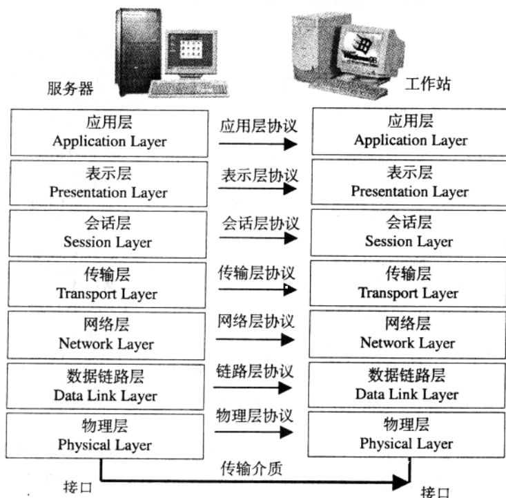
图 1-5 网络层次化结构模型
