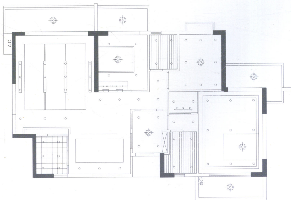
▲天花布置图
