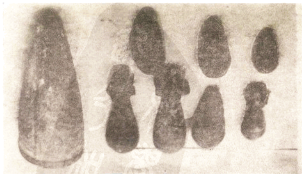
故县刘伯承铁厂铸造的部分 60、82 迫击炮弹壳
