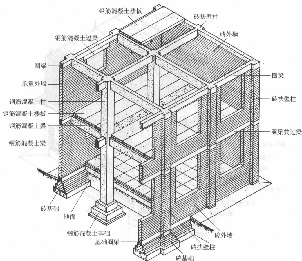
图 1-7 内框架承重结构建筑
