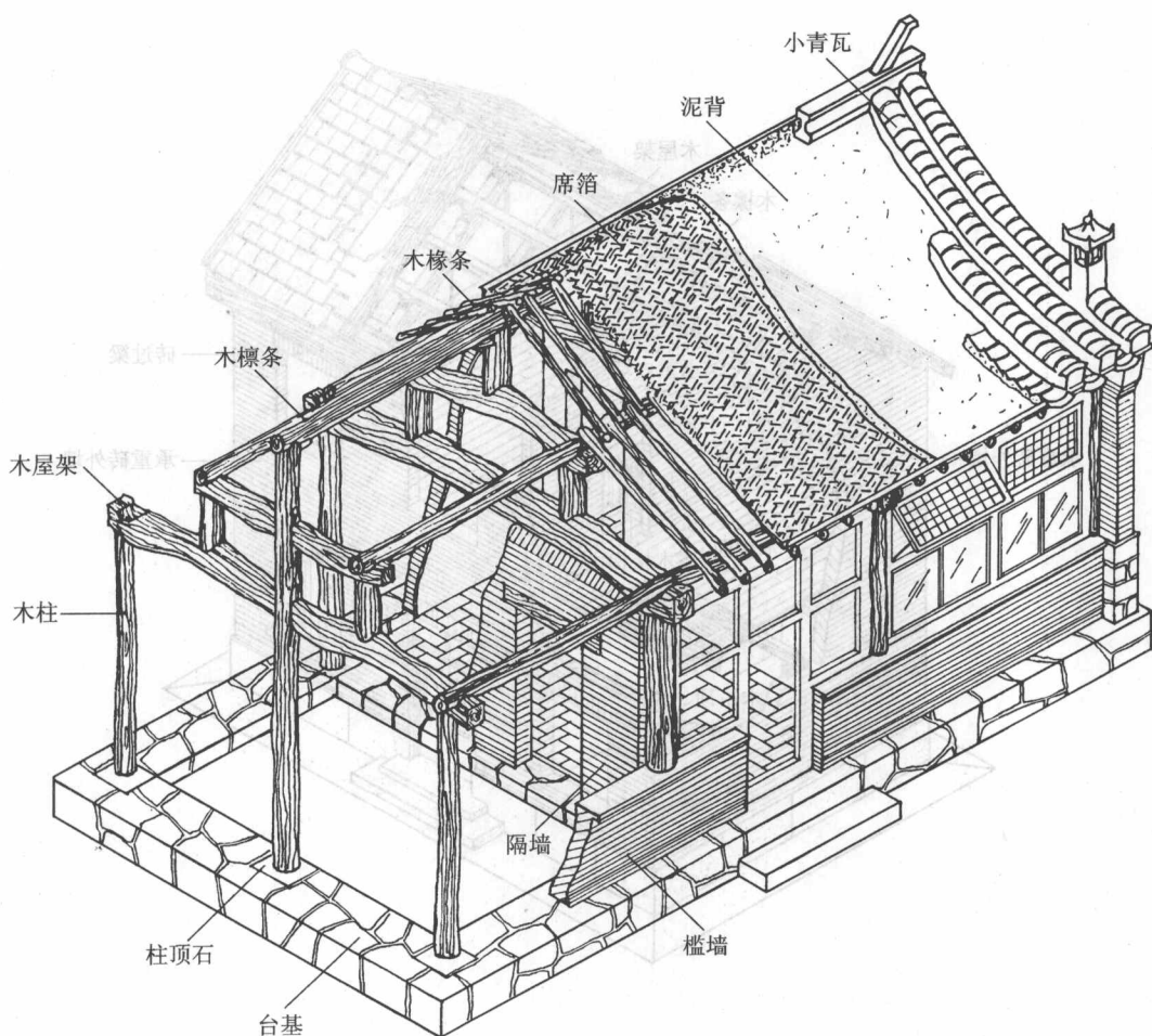
图 1-3 木结构建筑
