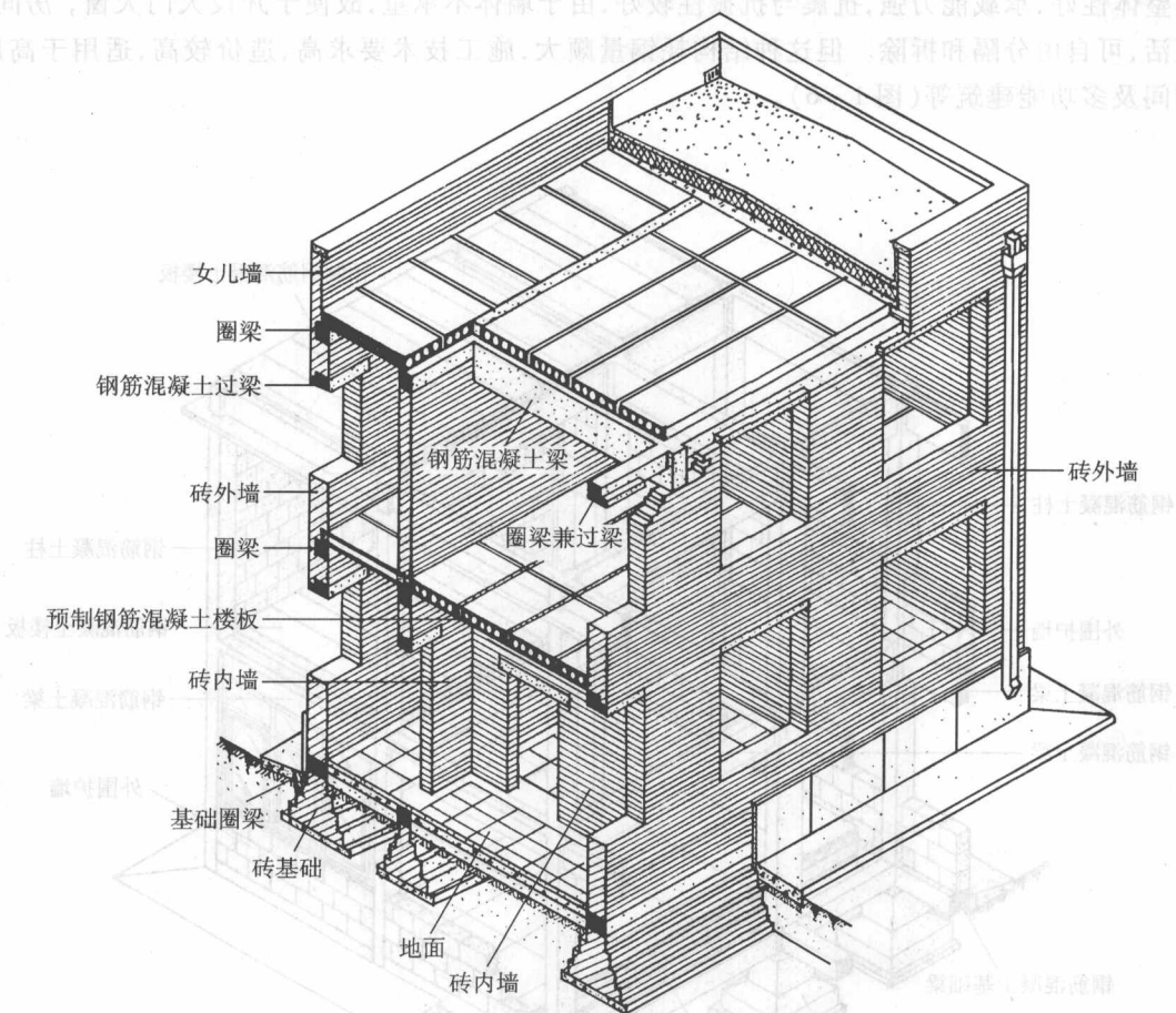
图 1-5 砖混结构建筑
