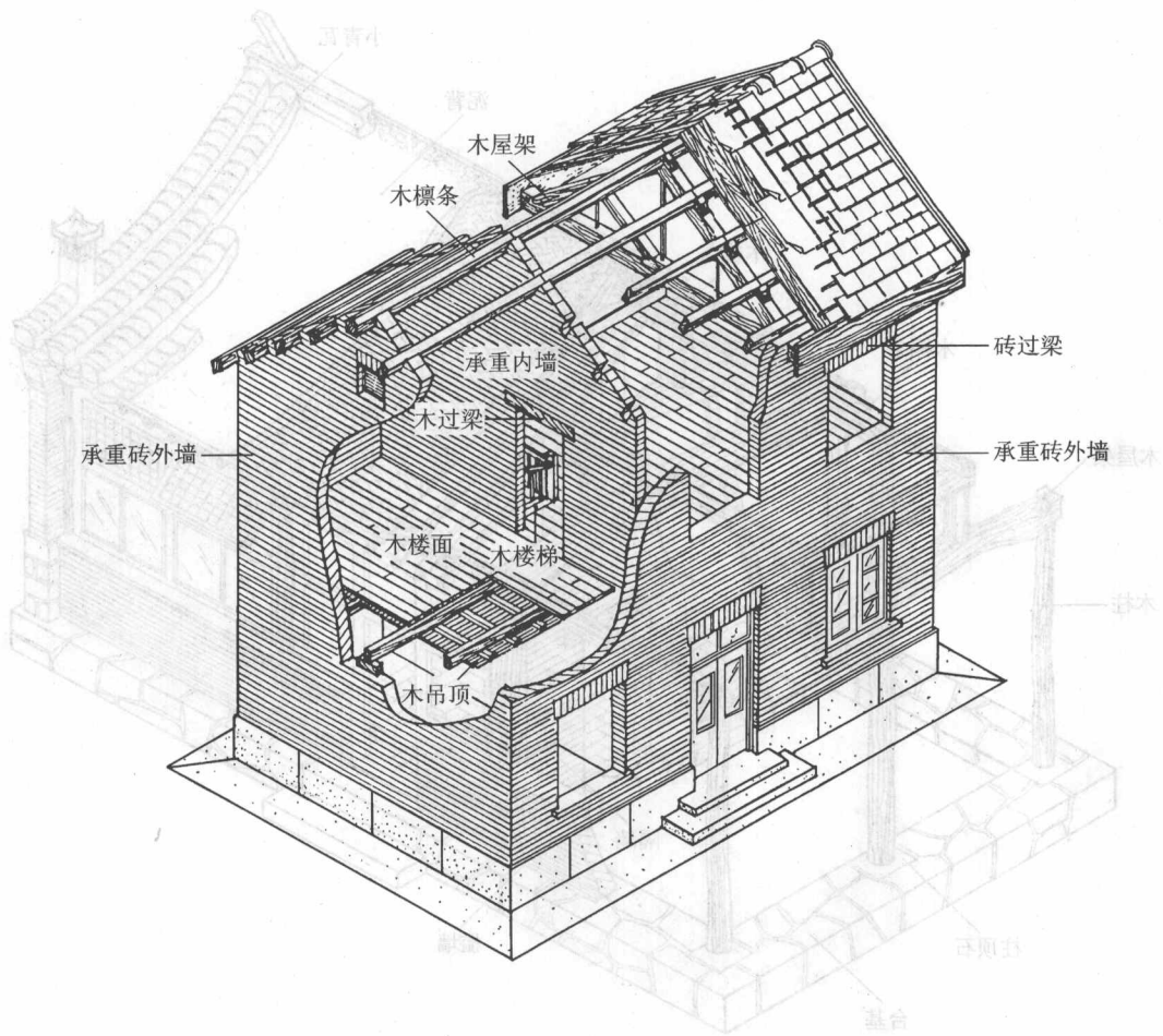
图 1-4 砖木结构建筑
