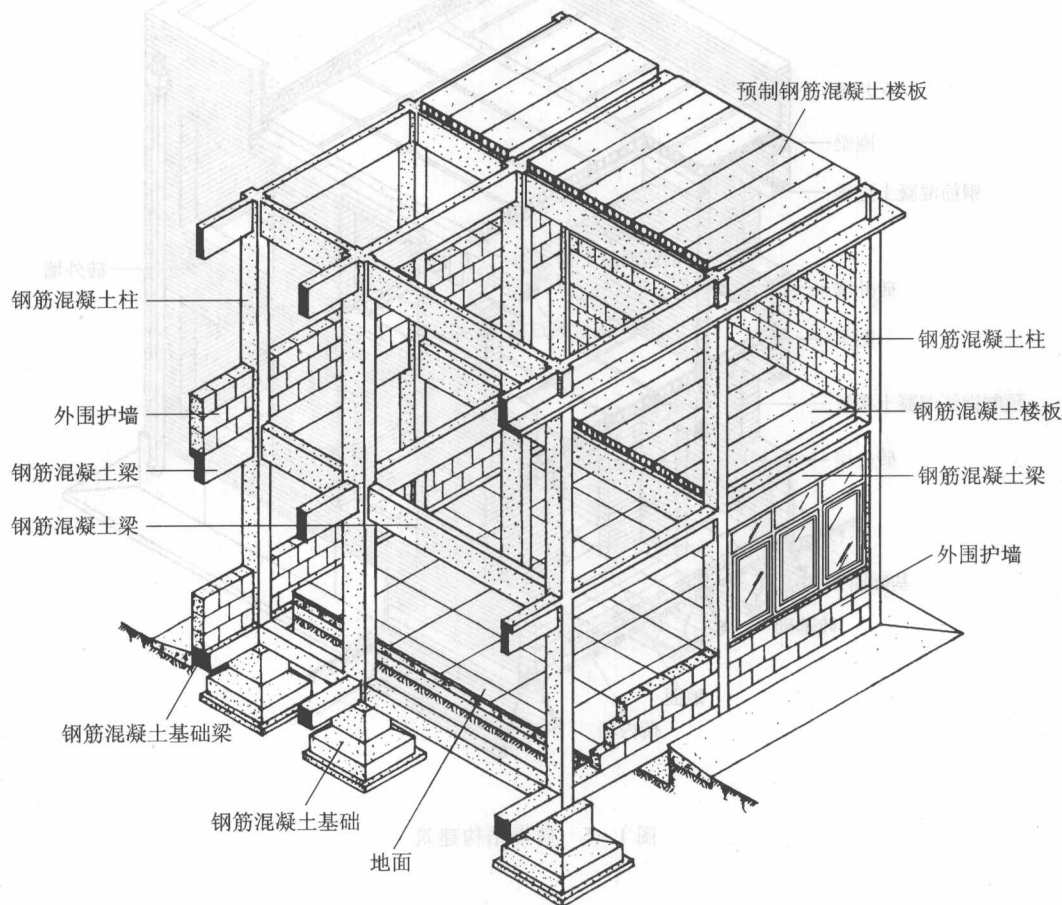
图1-6 钢筋混凝土全框架承重结构
