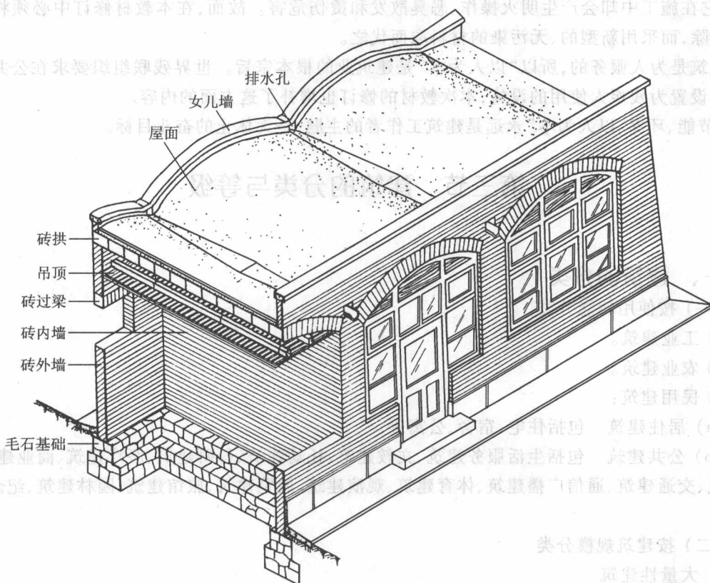
图 1-2 砖石结构建筑
