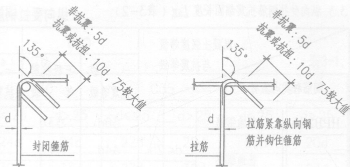
图6-1 梁、柱、剪力墙箍筋和拉筋弯钩构造
