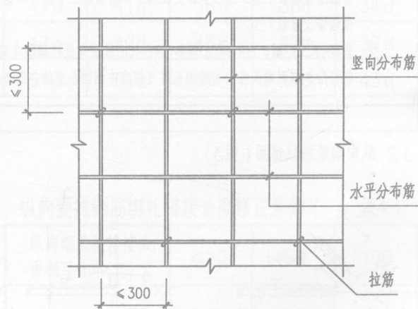
图2-3 剪力墙分布钢筋间距
