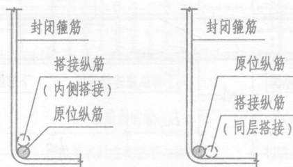
图7-2 封闭箍筋转角位置 (转角处无弯钩)
