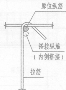
图7-3 拉筋弯钩位置
