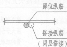
图7-4 箍筋平直段位置
