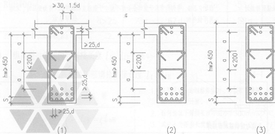
图2-1 梁纵向钢筋间距
