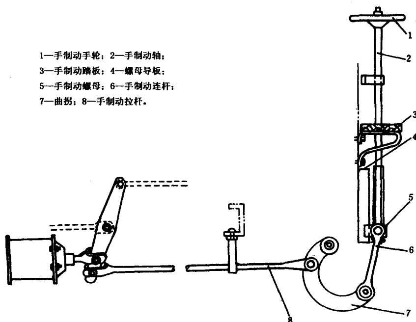
图 8-4-6 螺旋式手制动机
