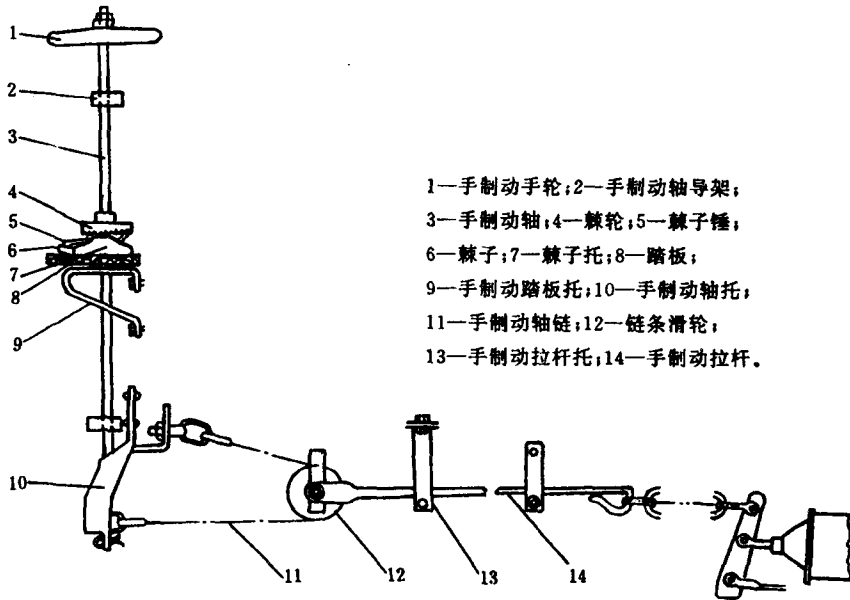
图 8-4-1 固定轴链条式手制动机
