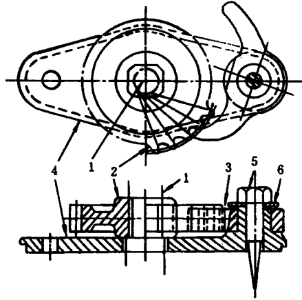
图 8-4-4 手制动轴防缓器之二
