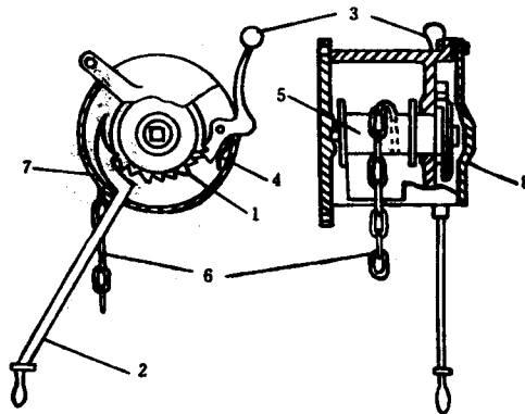
图 8-4-5 棘轮式手制动机
