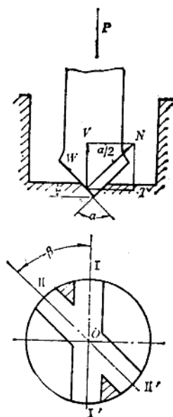
图 2-1 冲击转动式凿岩的动作原理
