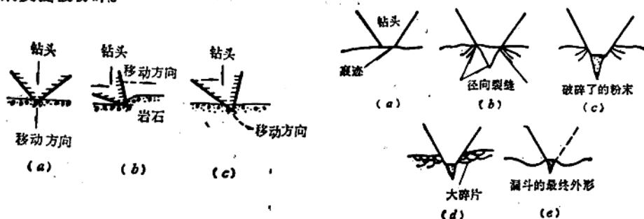
图 1-1 机械凿岩
