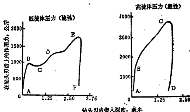
图 1-4 石灰岩的作用力-钻进深度曲线
