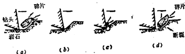
图 1-5 多刃旋转钻头的切削顺序
