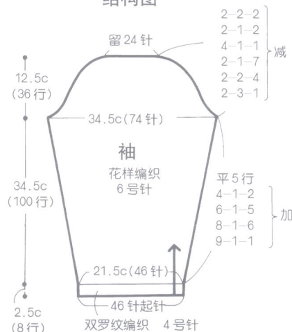
结构图
