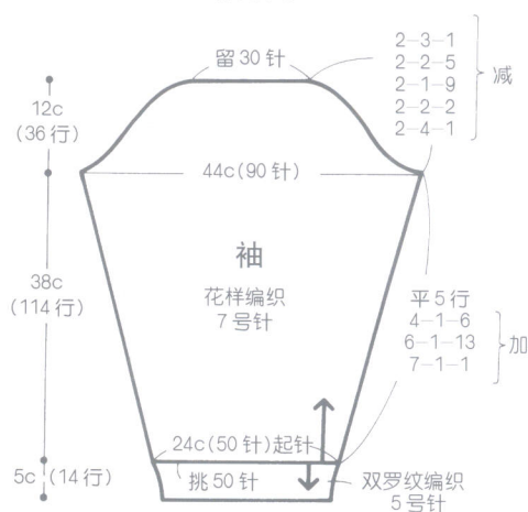
结构图
