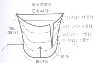
领结构图
