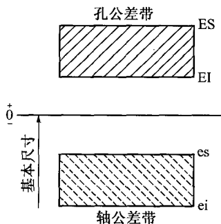
图 2-3 尺寸公差带图
