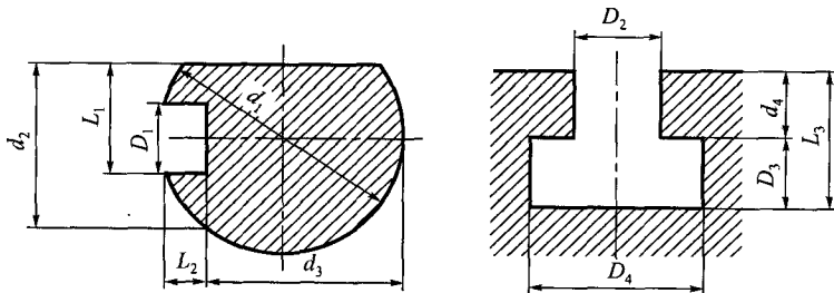
图 2-1 孔和轴
