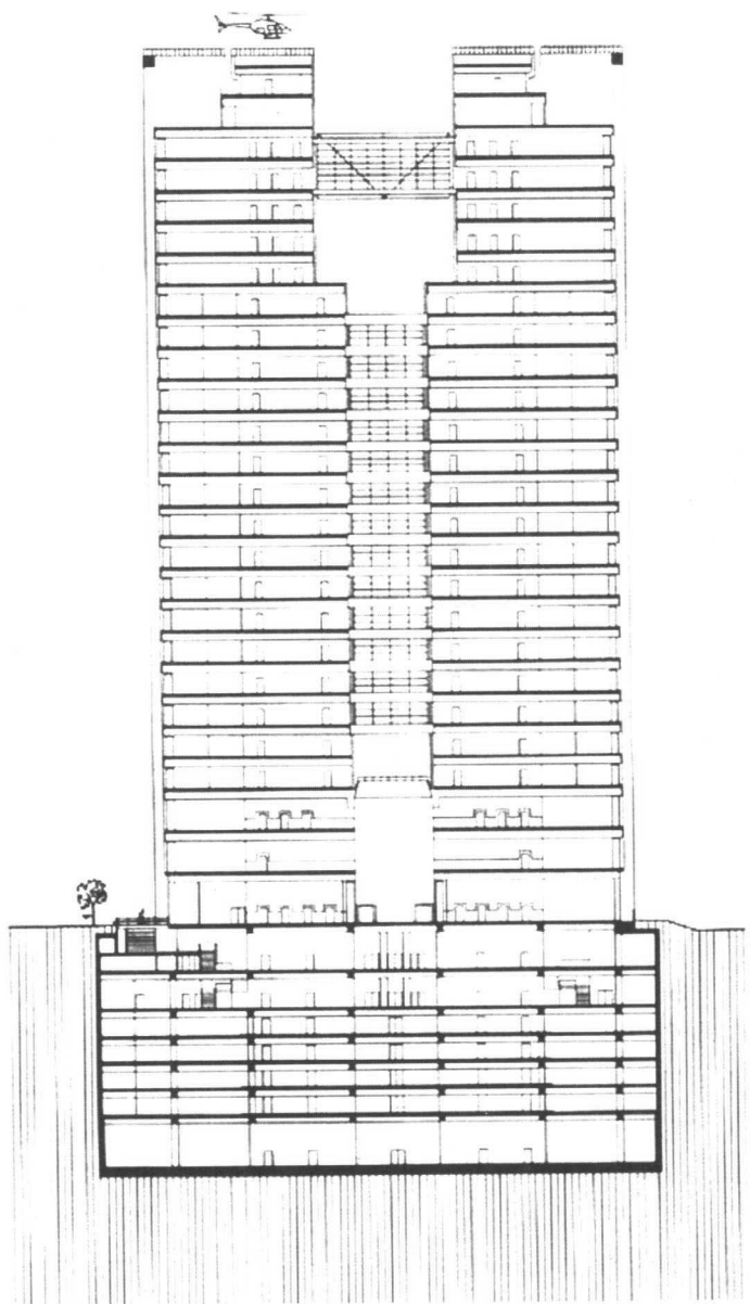
剖面图
