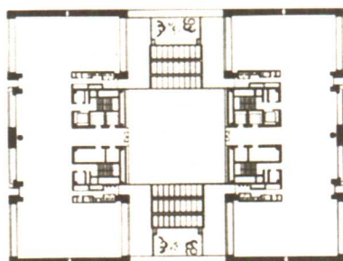
平面图
