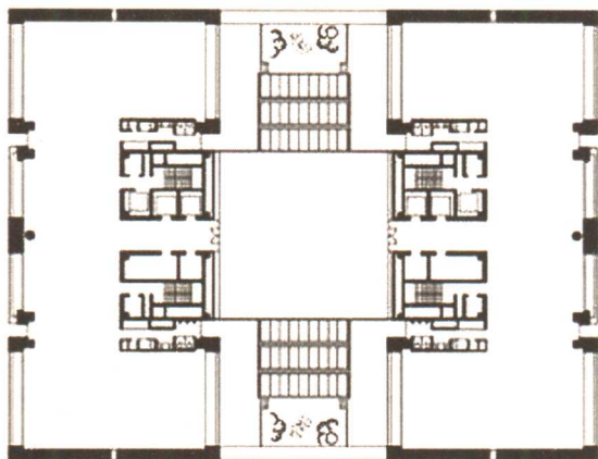
平面图
