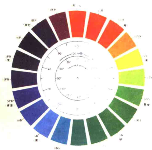
↑ 图 2-3 蒙赛尔色相环
