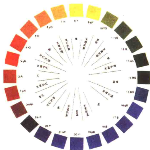
↑ 图 2-5 P.C.C.S 表色系
