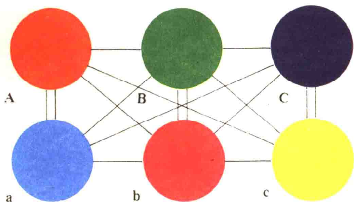
↑ 图 2-1 光的三原色与物体的三原色
