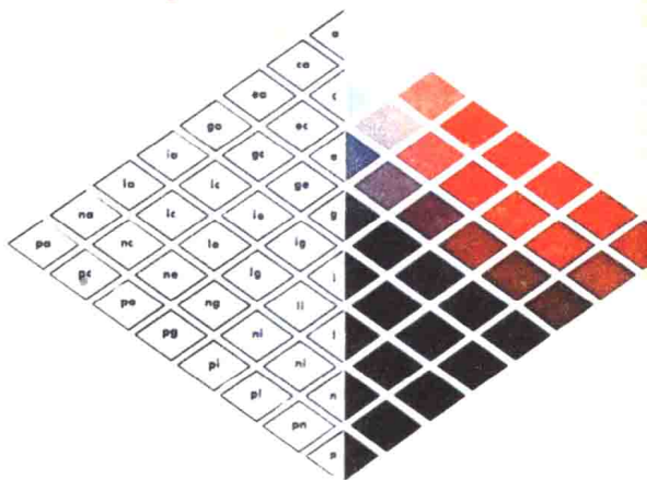
↓ 图 2-2 色彩的三属性示意图
