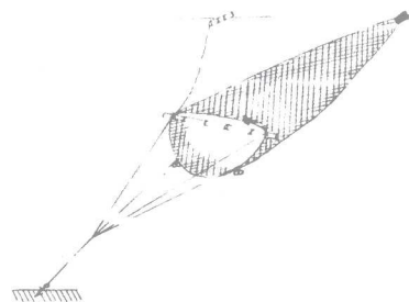
单碇张网作业示意图
