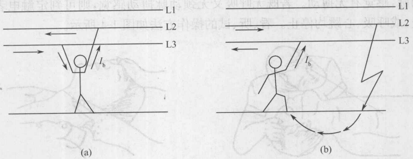
图 1-2 两相触电
