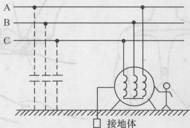
图 1-10 三相用电保护接地
