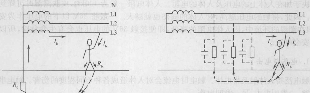
图 1-1 单相触电
