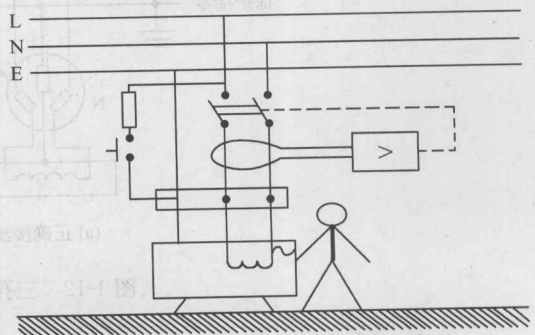
图 1-11 电流型漏电保护器
