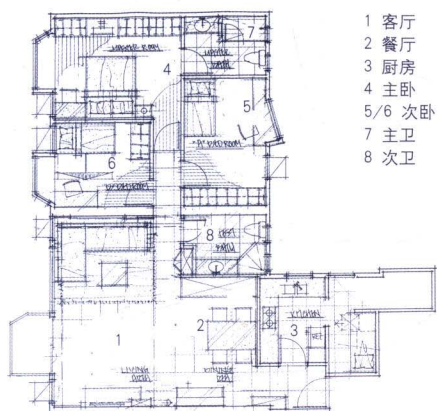
平面图
