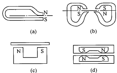
图 1-6 制动元件的结构形式
