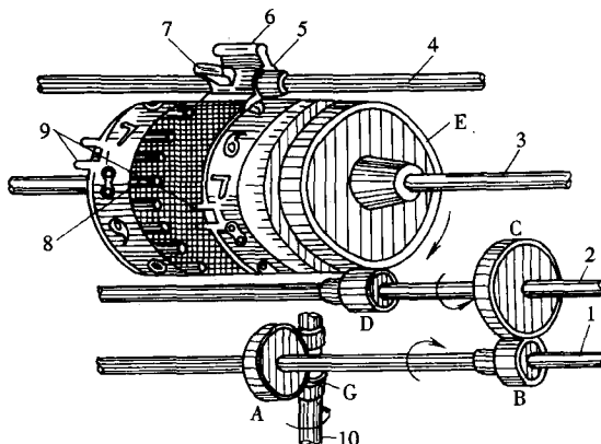
图 1-11 字轮式计度器结构
