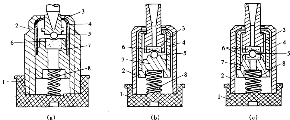
图 1-8 钢珠宝石轴承结构
