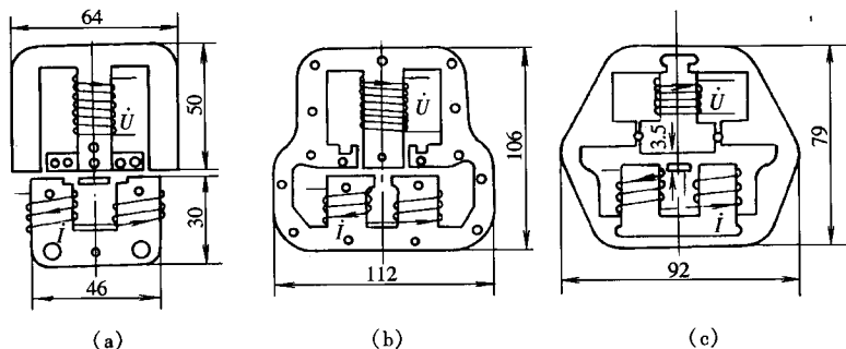
图 1-5 切线式驱动元件的结构形式
