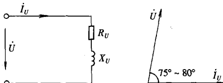
图 1-2 电压线圈的等值电路图和相量图
