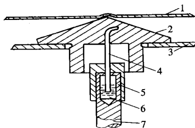
图 1-7 上轴承结构
