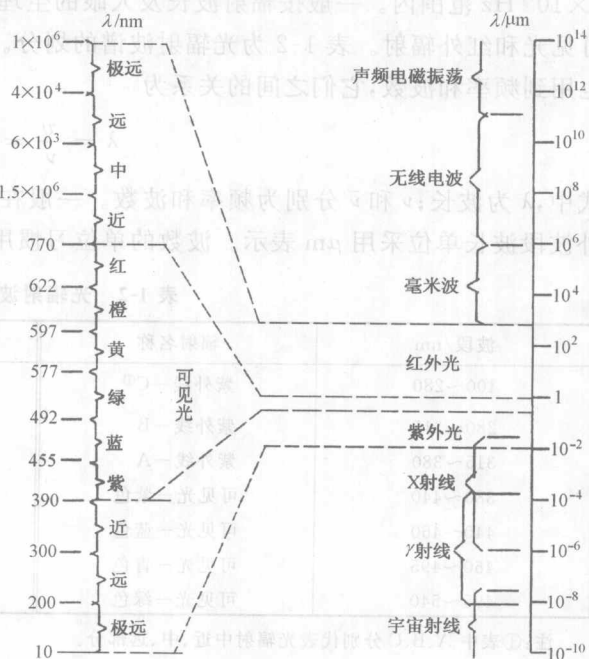
图 1-1 电磁辐射波谱
