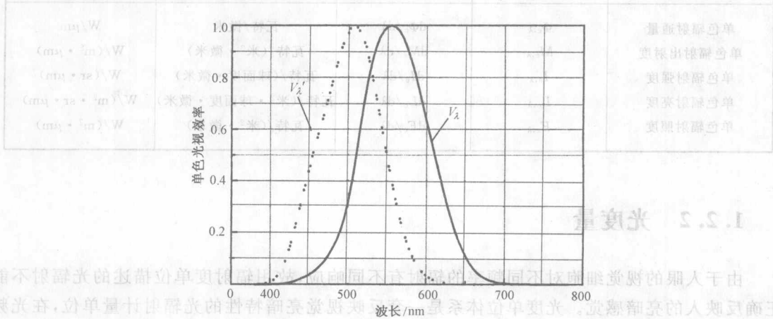
图 1-3 光谱光视效率曲线
