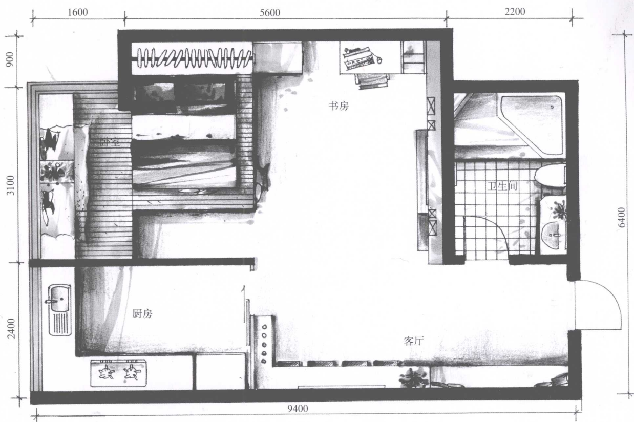
户型平面图
