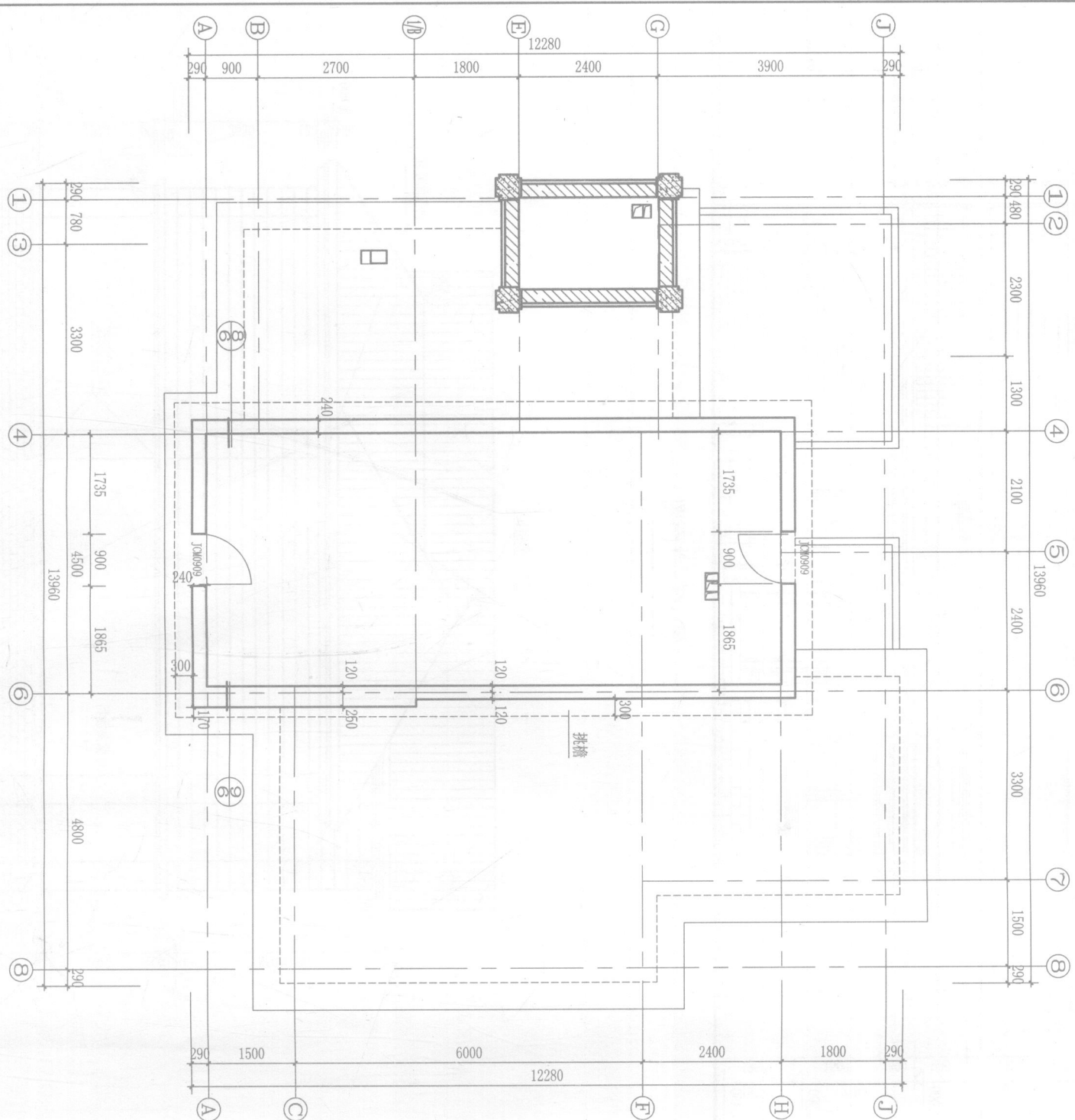
夹层平面图
