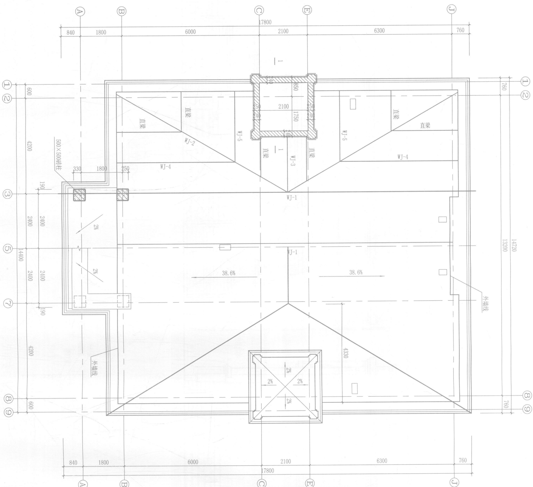
屋顶平面图
