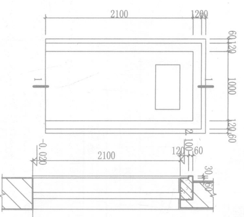
车库门口装饰大样
