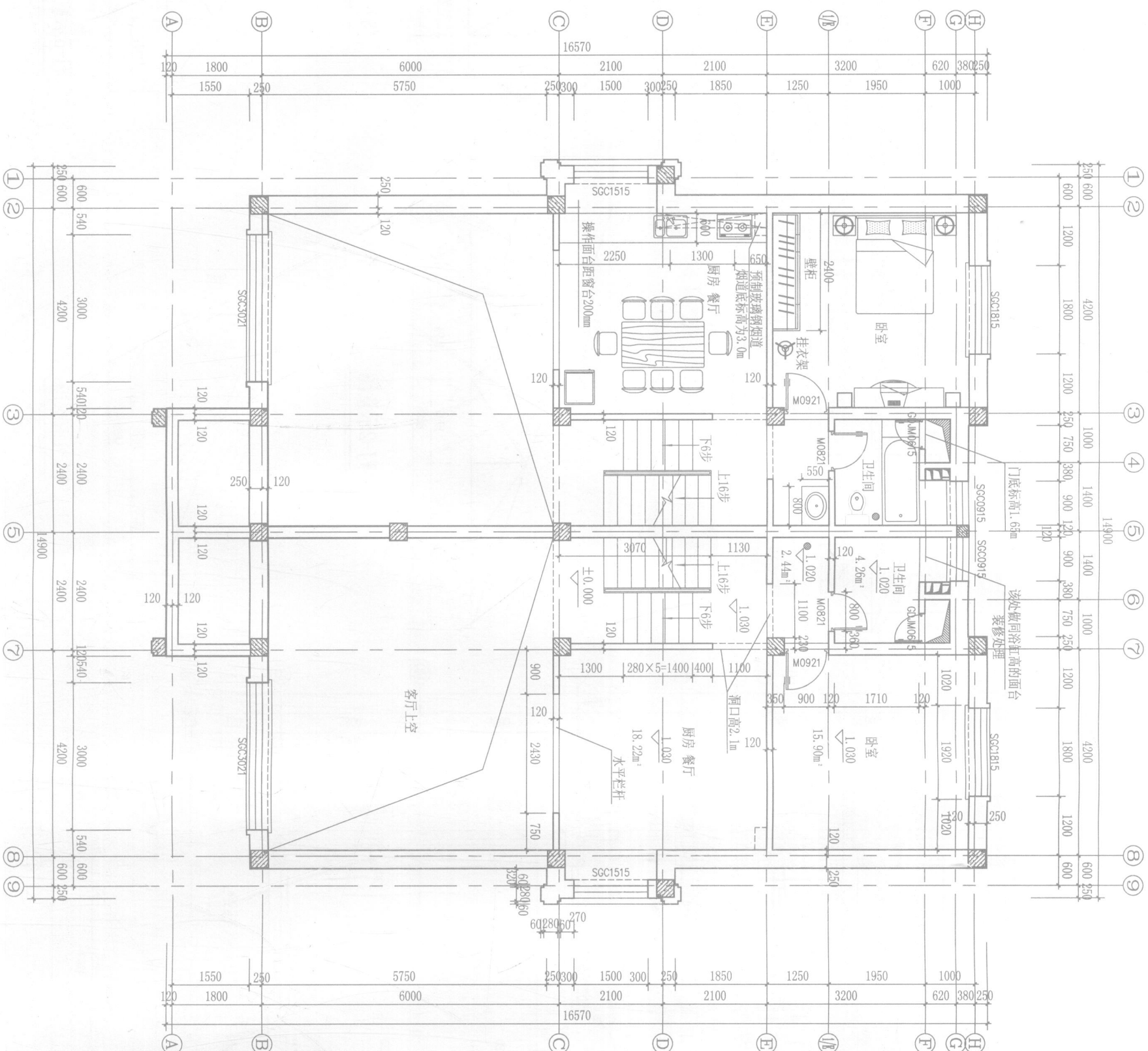
夹层平面图
