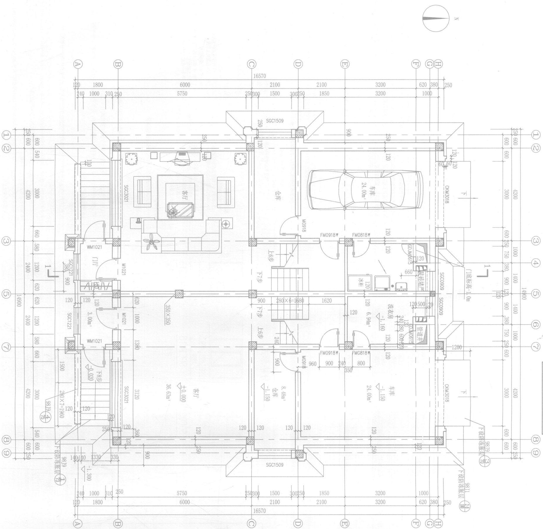
首层平面图
