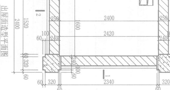
1 出屋面造型平面图
