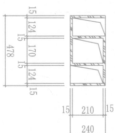
卫生间风道示意图
