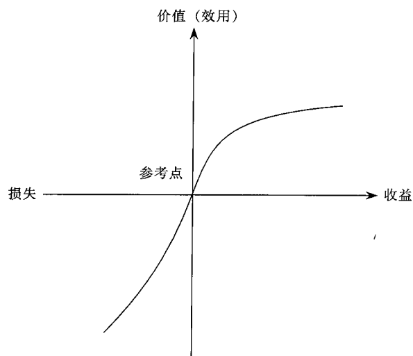
图1 价值函数
