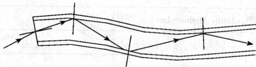
图 1-6 全反射光纤
