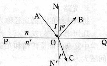
图 1-4 光的反射与折射现象
