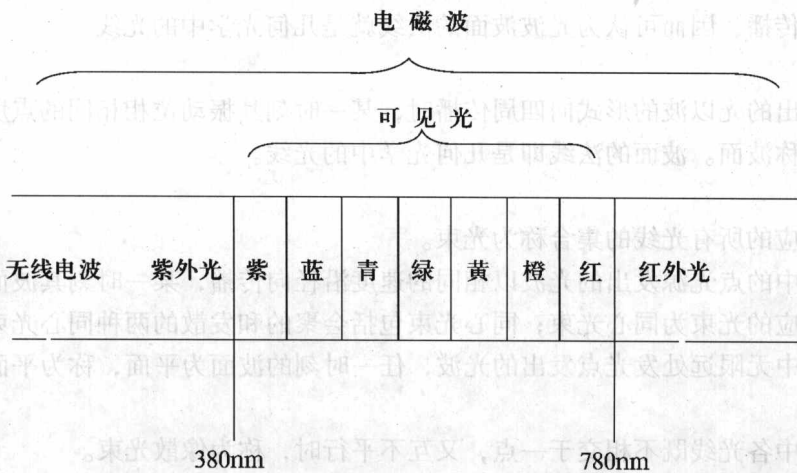
图 1-1 电磁波的不同波长区域
