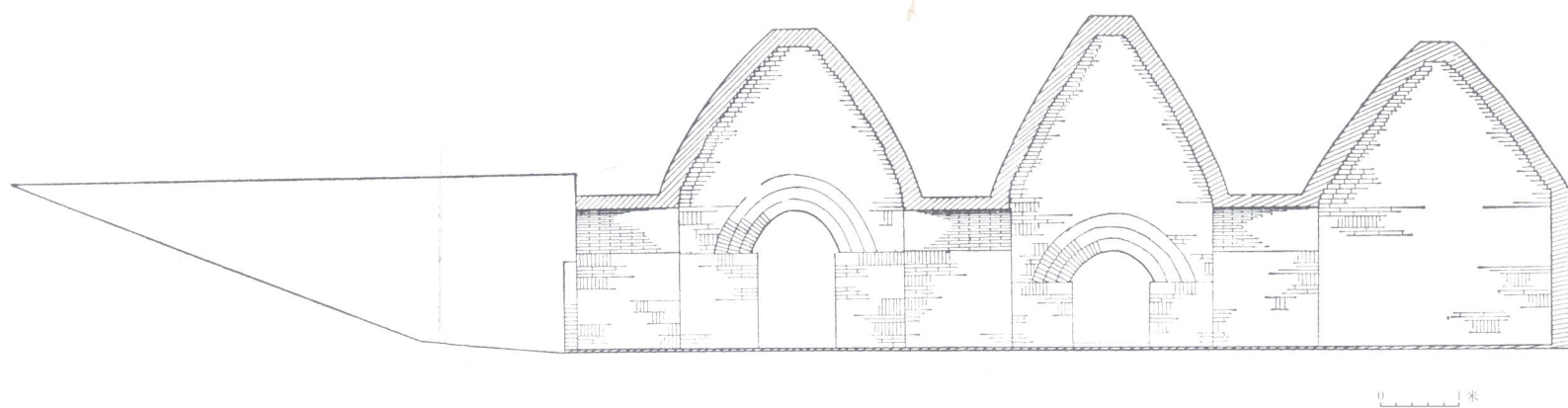
图4 墓葬纵剖面图
