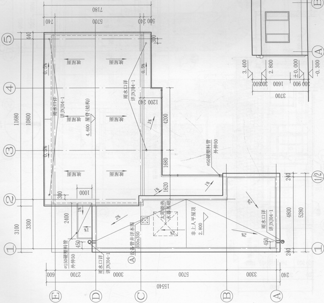
屋顶平面图
