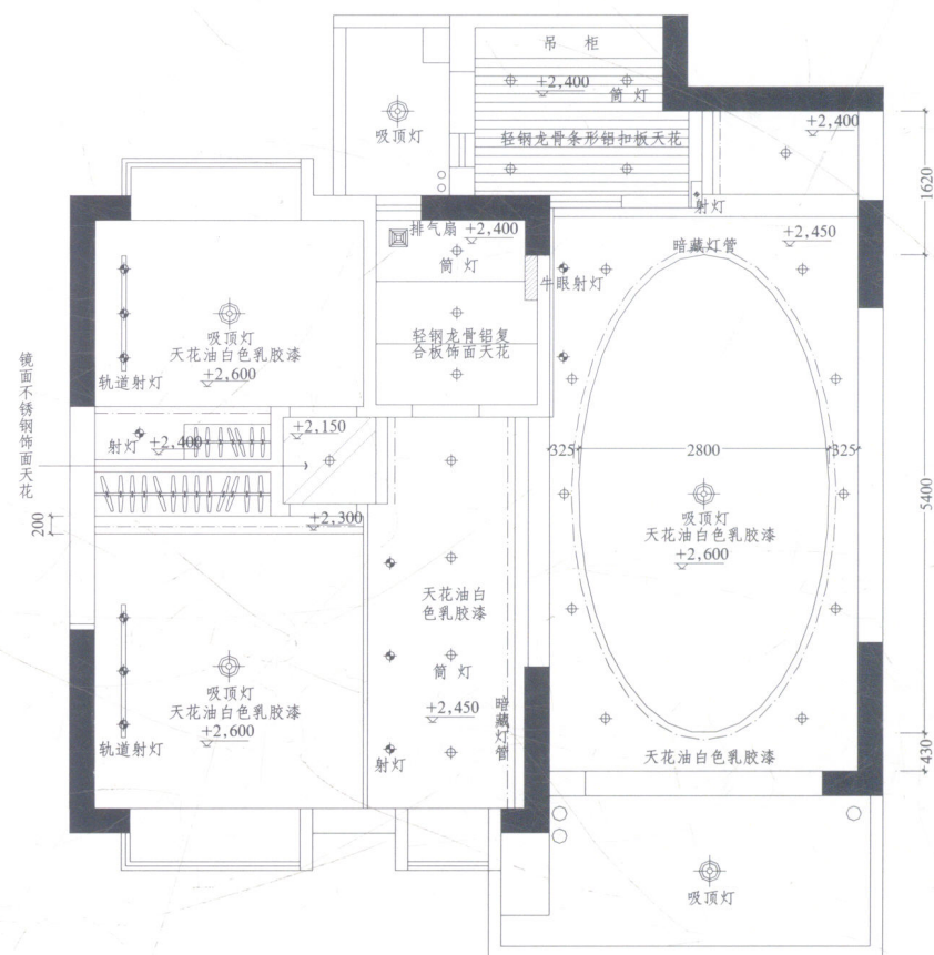
◆天花布置图
