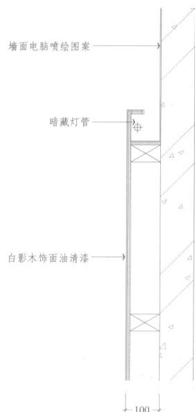
◆主卧室立面图11-a节点详图
