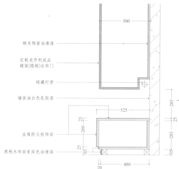
◆主卧室立面图10-a节点详图
