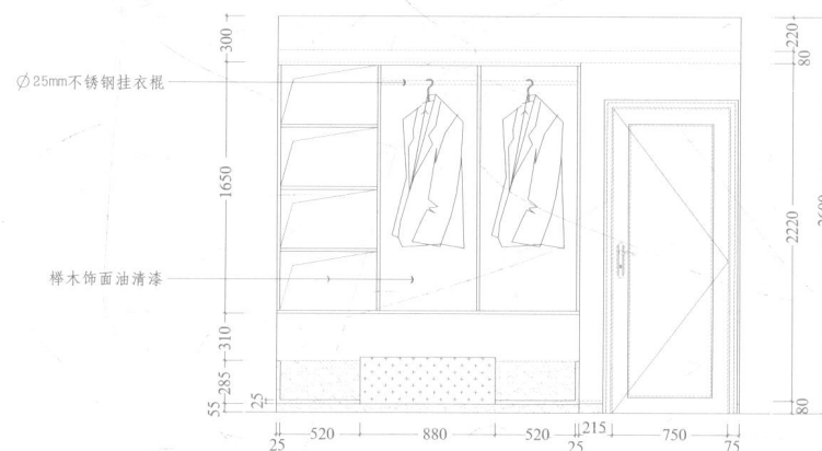
◆主卧室立面图10衣柜内部结构图
