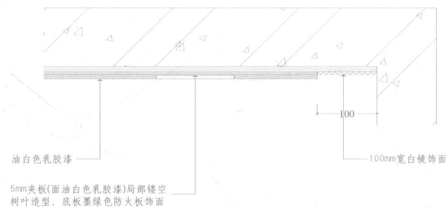
◆ 客厅立面图 1-b 节点详图
