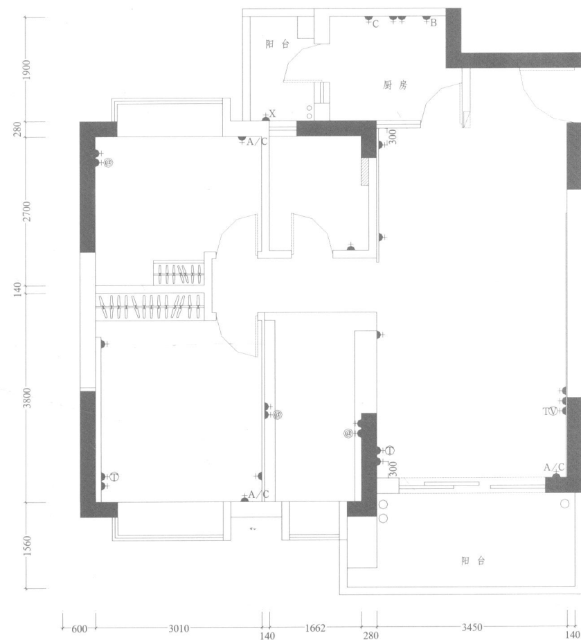
◆ 插座布置图
