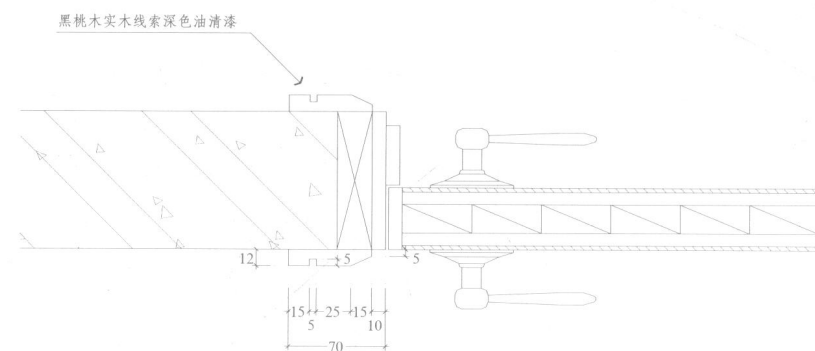
◆主卧室立面图10-b节点详图
