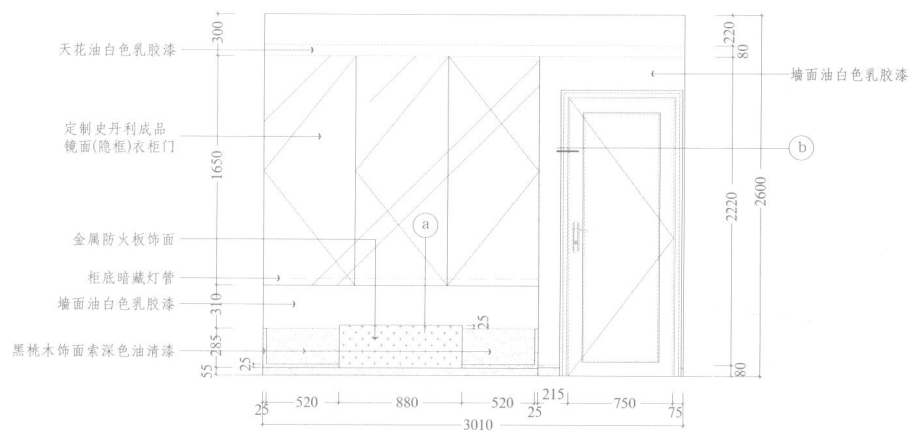
◆主卧室立面图10
