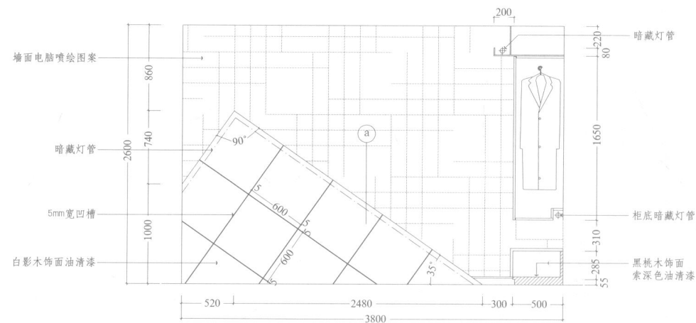
◆主卧室立面图11
