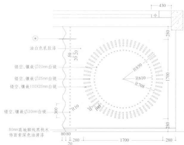
◆ 客厅立面图 1-a 大样图
