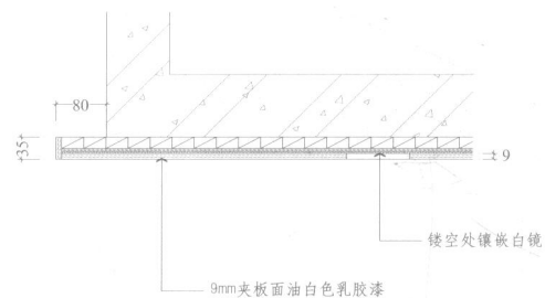
◆ 客厅立面图 1-a 节点详图 *
