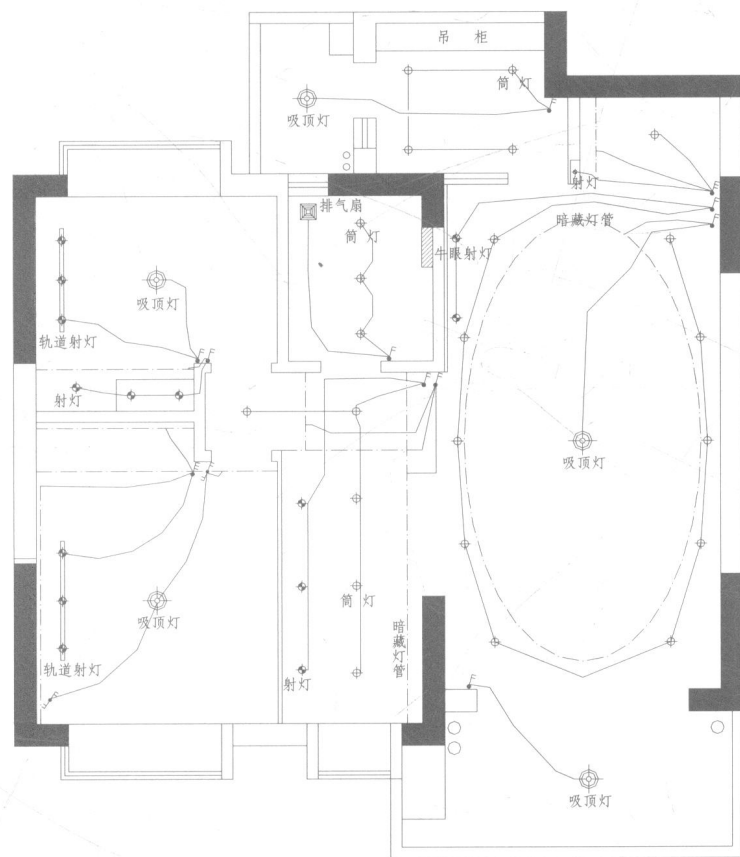
◆ 灯具开关布置图
