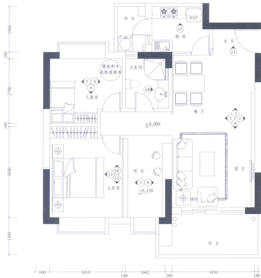
◆平面布置图
