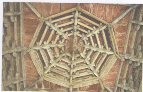
10-7 山西长治关帝庙大殿内藻井（明代）
