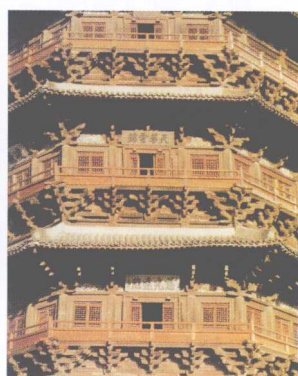
9-8 山西应县佛光寺木塔细部（辽，应县城西北佛光寺内）
