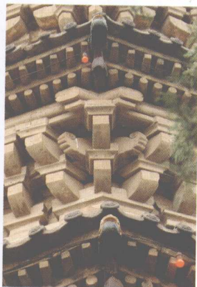
6-5 山西潞城原起寺宋塔局部
