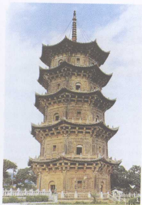
6-7 福建泉州开元寺塔（南宋嘉熙二年至淳祐十年，1238-1250年，泉州市）
