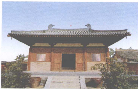
1-1 山西五台山南禅寺大殿（唐建中三年，782年，五台县城阳白乡李家庄村）
