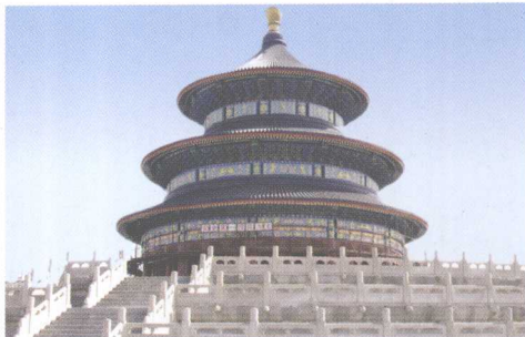
3-2 北京天坛祈年殿（明永乐十八年，1420年，崇文区）
