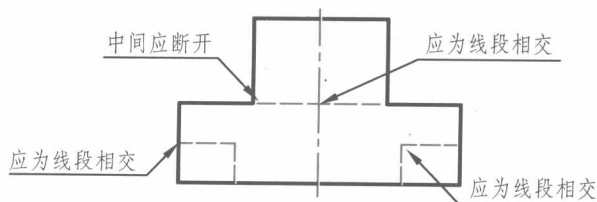
图 1-8 点画线、虚线、实线交接画法
