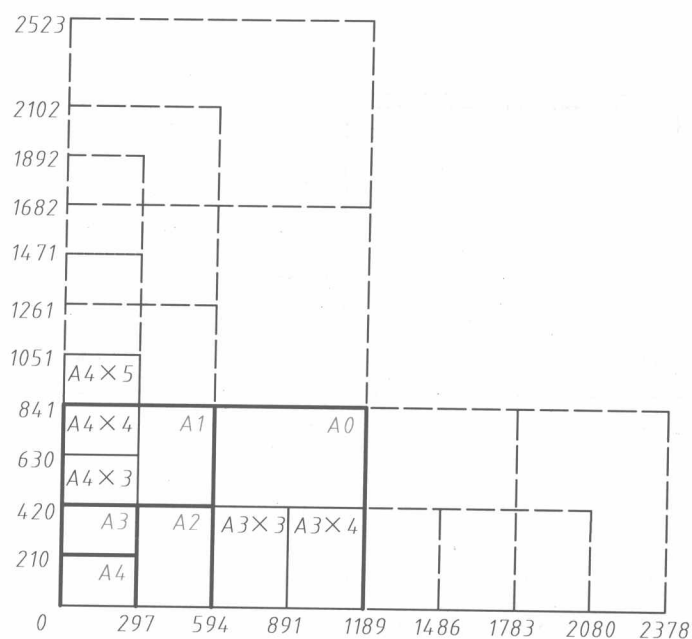
图 1-1 图纸幅面
