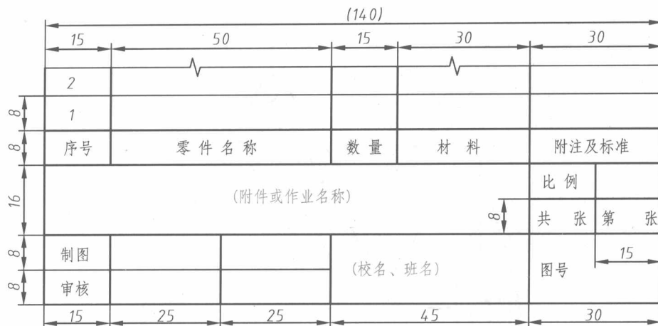
图 1-5 装配图的标题栏与明细栏
