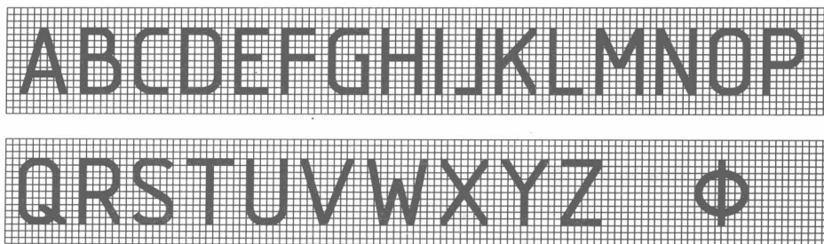
B 型小写直体拉丁字母和希腊字母 \phi
