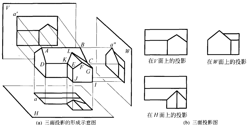
图 1-4 正投影的基本性质
