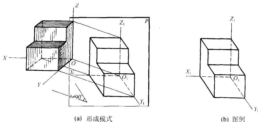
图 1-11 斜轴测图
