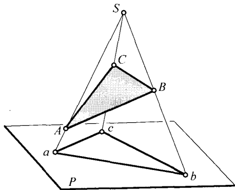
图 1-2 中心投影法
