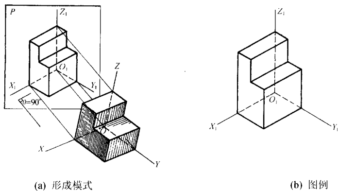
图 1-10 正轴测图
