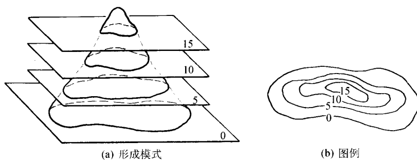
图 1-13 标高投影图
