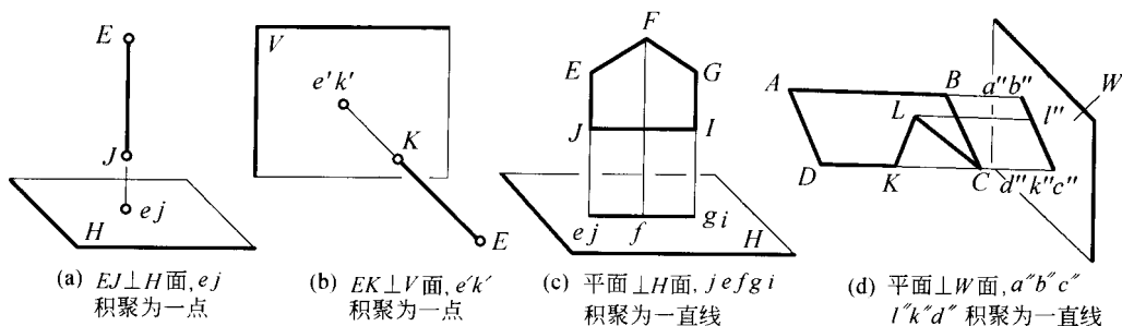
图 1-6 正投影的基本性质——积聚性
