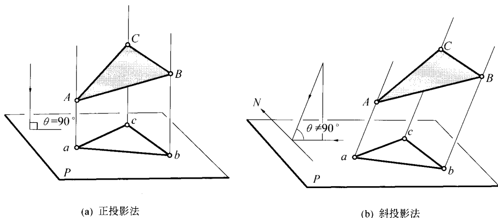
图 1-3 平行投影法
