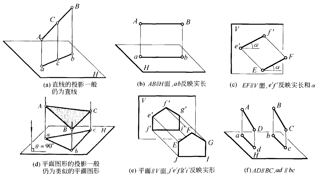
图 1-5 正投影的基本性质——不变性
