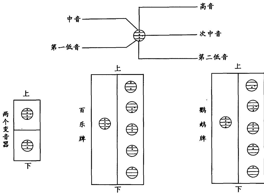
图6 左手键钮变音器
