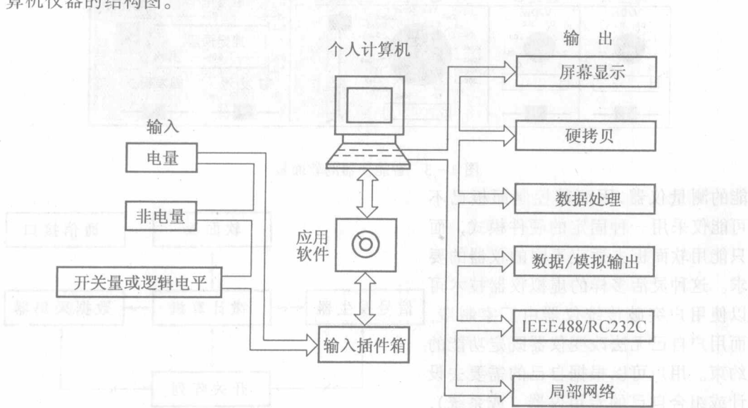
图 1-2 个人计算机仪器 (PCI) 的结构图
