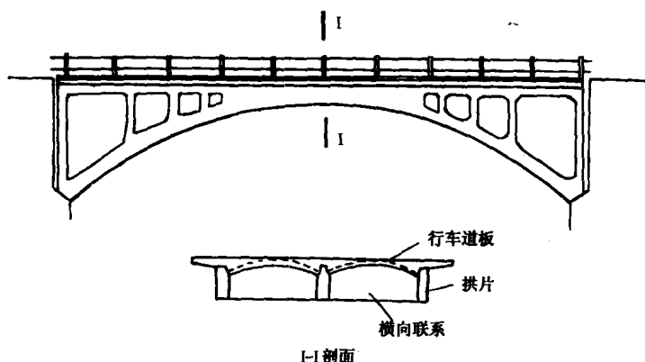
图 1-1-8 拱片桥
