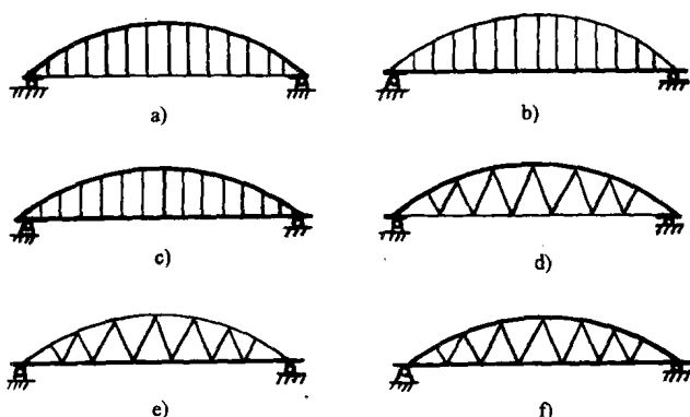
图 1-1-6 无推力的组合体系拱
