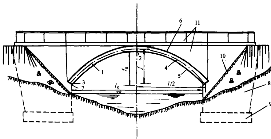
图 1-1-4 实腹拱桥
