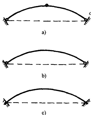
图 1-1-5 拱圈(肋)的静力图式
