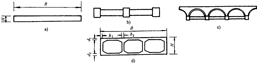
图 1-1-9 拱的横截面型式
