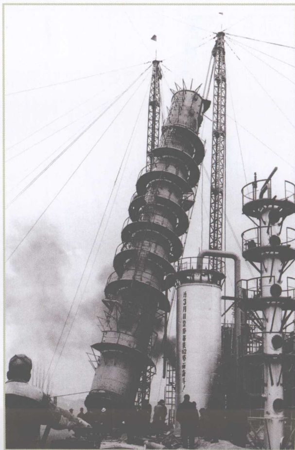
1958年兰州炼油厂减压塔进入最后吊装阶段
