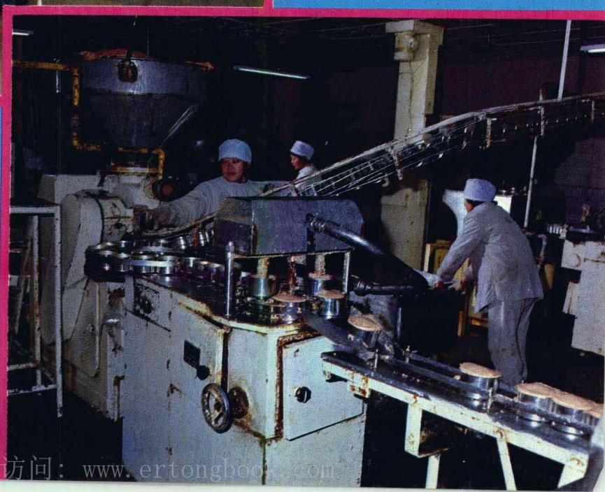
蚌埠肉联厂午餐肉罐头生产流水线
