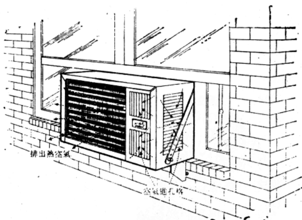
圖4．冷氣機室外部分的吸氣、排氣情形
