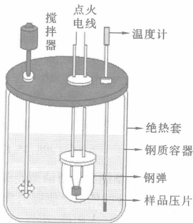
图 1-1 弹式量热计示意图
