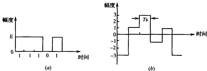
图 1-3 二进制与多进制数字信号
