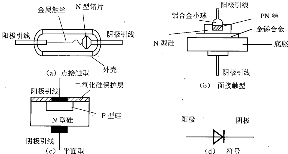
图 1-10 半导体二极管的结构和符号
