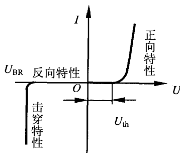
图1-11 硅二极管的伏安特性曲线
