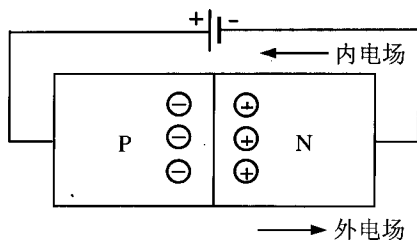
图 1-8 外加正向电压
