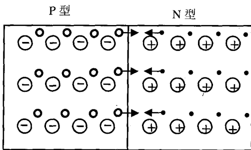
图 1-6 载流子的扩散
