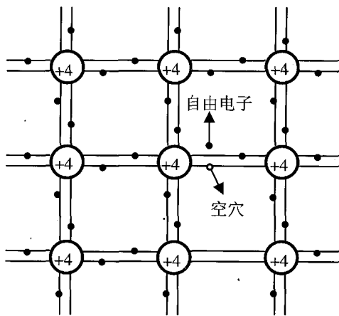
图 1-3 半导体中的两种载流子
