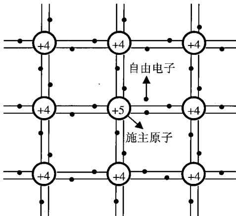
图 1-4 N 型半导体二维结构示意图
