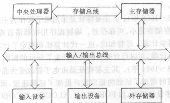
图 1.2 计算机硬件结构
