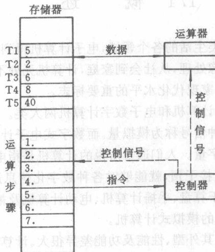
图 1.1 计算机模型
