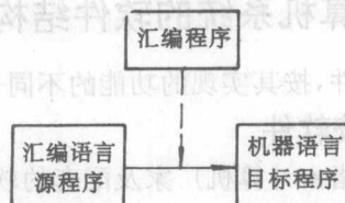
图 1.3 汇编过程
