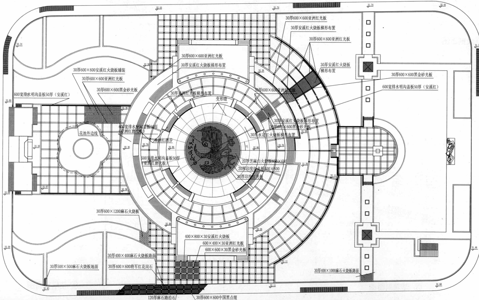
铺装总平面图
