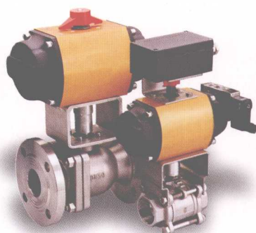
精小型气动O型切断球阀
