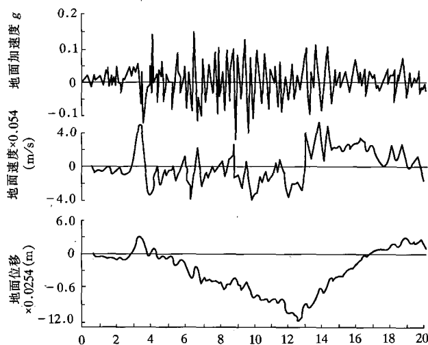
图 1-5 地面运动的加速度、速度、位移
