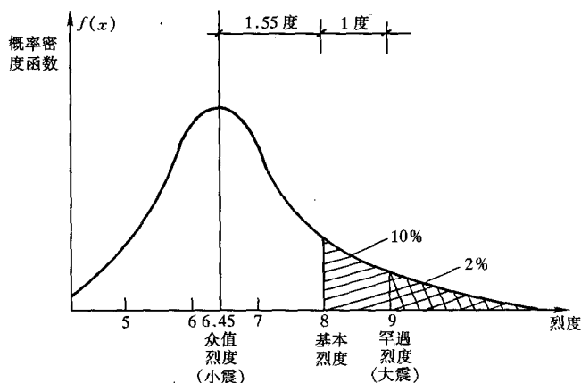
图 1-8 三种烈度含义及其关系
