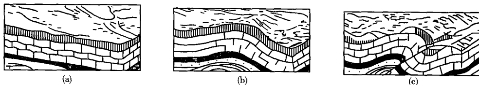
图 1-2 岩层的变形与破裂
