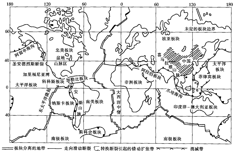
图 1-1 板块分布图
