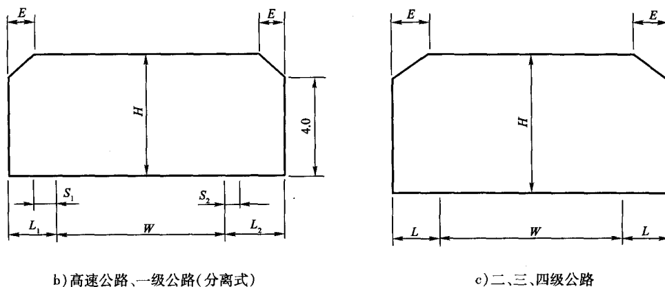
图 3.3.1 桥涵净空(尺寸单位:m)
