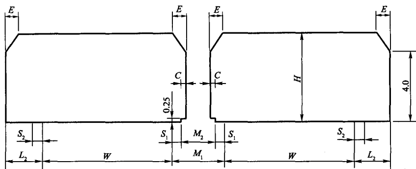
a) 高速公路、一级公路(整体式)
