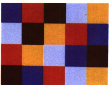
彩图 19 三原色与极色
