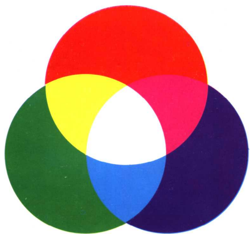
彩图 6 色光三原色与三间色
