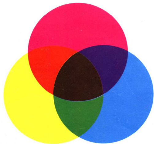
彩图 7 颜料三原色与三间色
