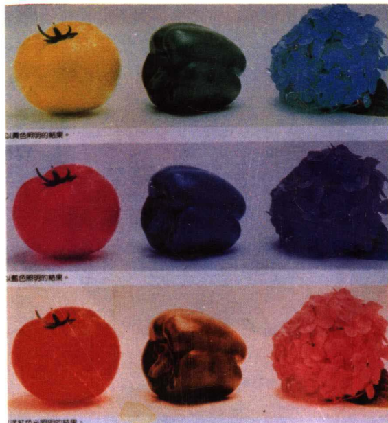
彩图 3 黄光、蓝光、红光照射下的物体色彩变化
