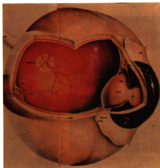
彩图 5 眼球解剖模型
