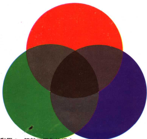
彩图 8 颜料三间色的混合
