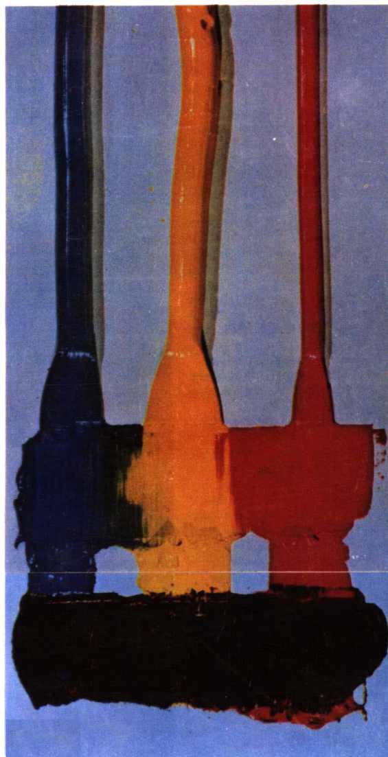
彩图 4 颜料三原色混合
