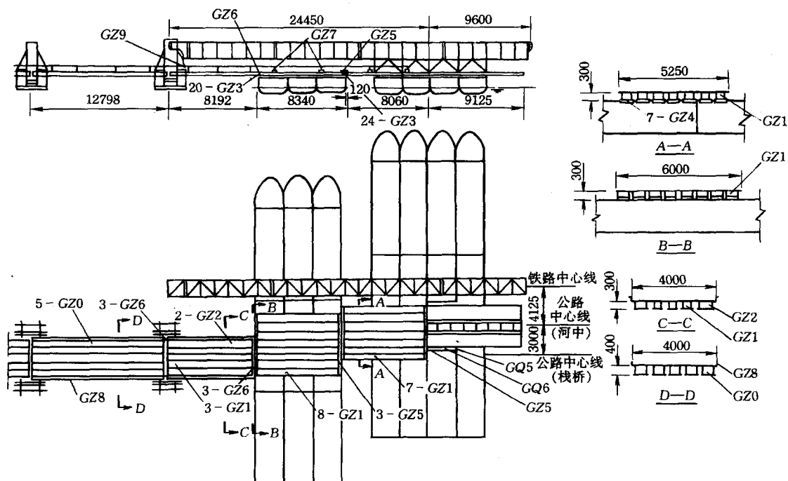
图 1—3 公路过渡部分(单位:mm)
