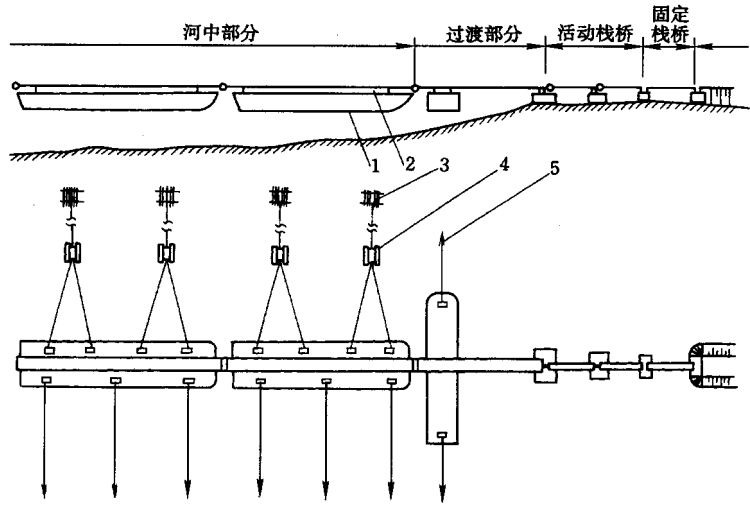
图 1—5 纵置式铁路浮桥
