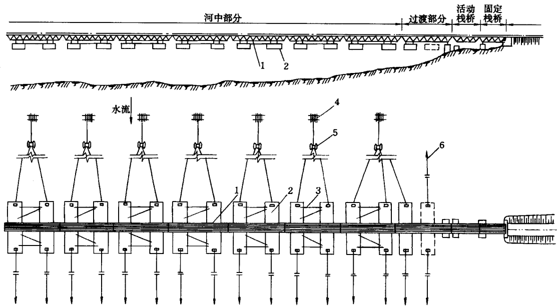
图 1—4 分置式铁路浮桥
