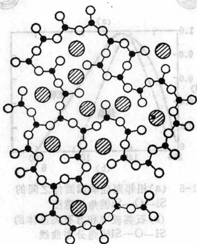
图1-4 无规则网络学说的钠硅酸盐玻璃结构模型
