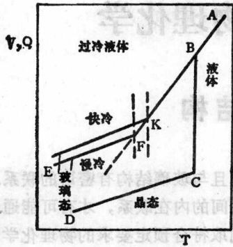
图1-1 物质内能与体积随温度的变化
