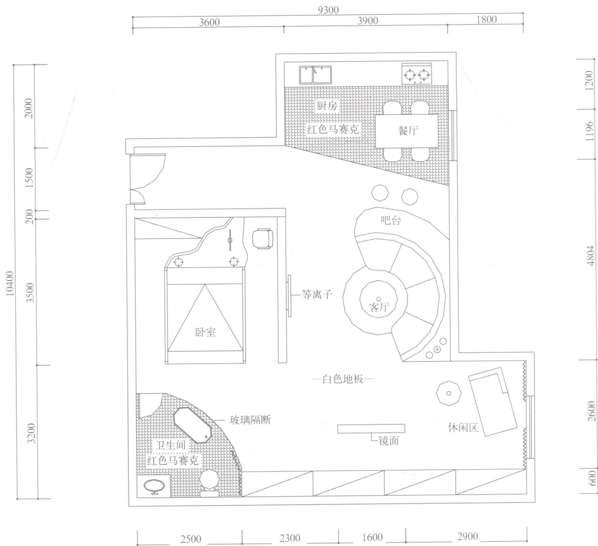
户型平面图
