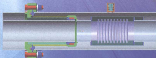
➡ 真空管道法兰连接结构简图
