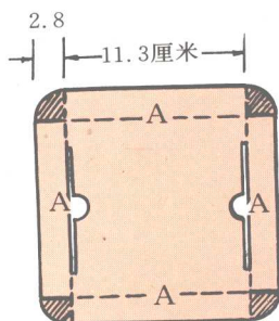
(1) 正方形盒盖展开图;
