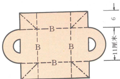
(3) 正方形盒身展开图 (B 比 A 短 3 毫米);
