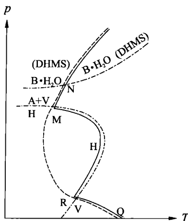
图 1-1b 向高压扩展的脱水熔融固相线
