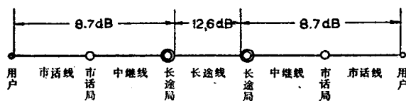
图 1.3 通信网的净衰减分配
